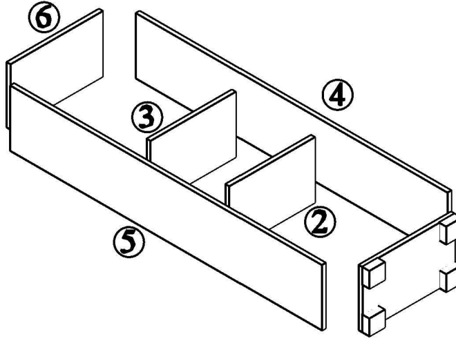
SABİT RAFLARLA SAĞ YAN VE SOL YANLARI MONTAJ EDİN ALT TABLAYI MONTAJ EDİN ÜST TABLAYA MONTAJ EDİN NOT. BU İŞLEMİ ÜRÜN YERDE YATAY İKEN YAPINIZ
