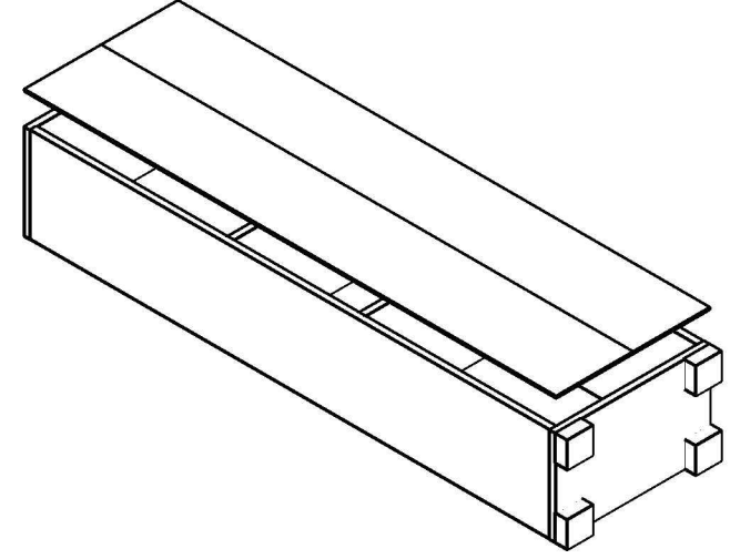
DOLABI GÜNTE YE GETİRİP ARKALIKLARI ÇAKINIZ NOT. BU İŞLEMİ ÜRÜN YERDE YATAY İKEN YAPINIZ
