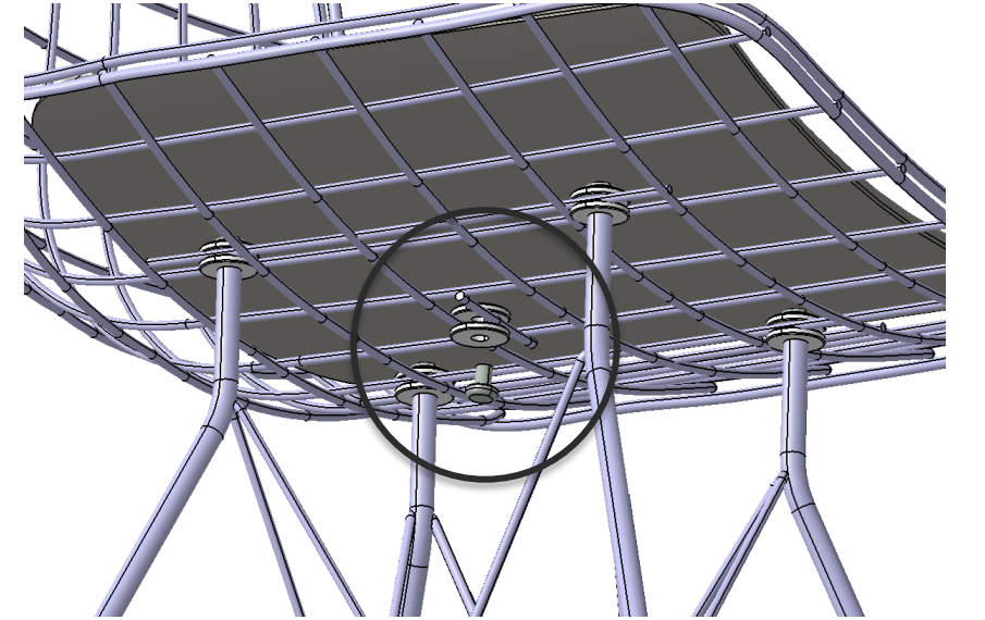
6. Döşemenin alttan bağlantı civatası takılarak montaj işlemi tamamlanır.
