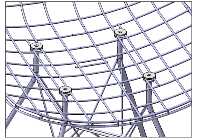
3. Pullardan sonra karkas ve tekrar pul yerleştirilir.
